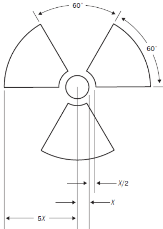
三叶形符号及以中心圆半径 x 为基础的各部分的比例
