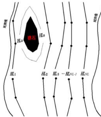
图 C-2 河床水下地形等高线
