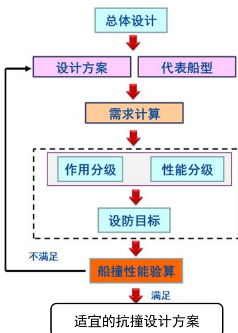
图 4.1.3 桥梁抗船撞设计流程
