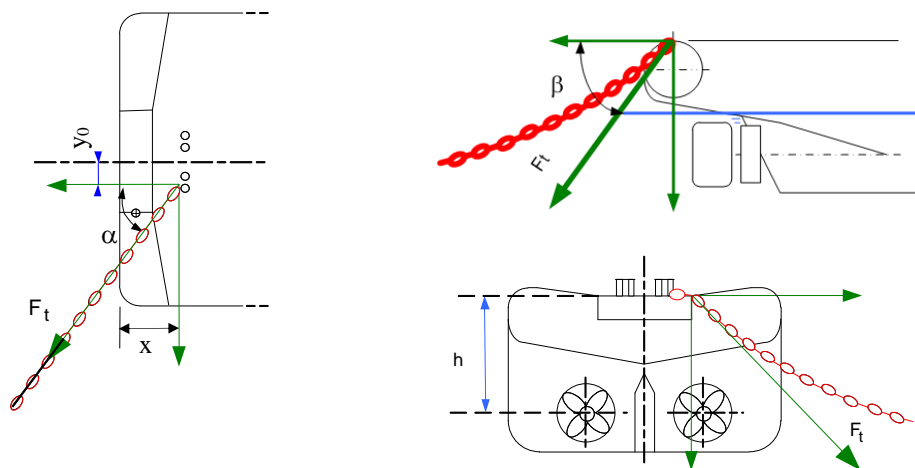
图 2.7.2 – 上图显示参数 \alpha , \beta , x , y 和 h 的预期意义。 F_t 表示缆绳承载张力的矢量。”
