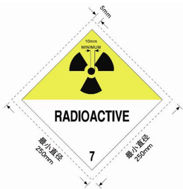
第 7 类放射性物质标牌
