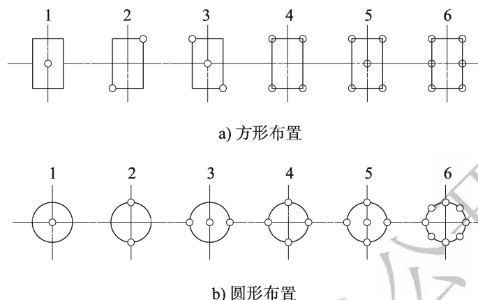
图 6.11.3 勘探钻孔布置图
