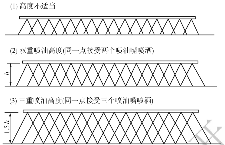
图 6-1 沥青洒布车喷油嘴的高度
