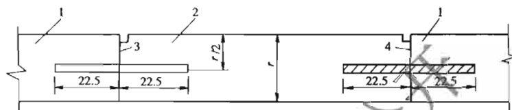
图 7.1.3-3 设置传力杆法(单位:cm)
