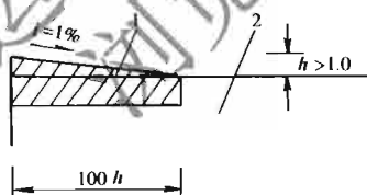
图 7.5.3 错台填补法示意图(单位:cm)
