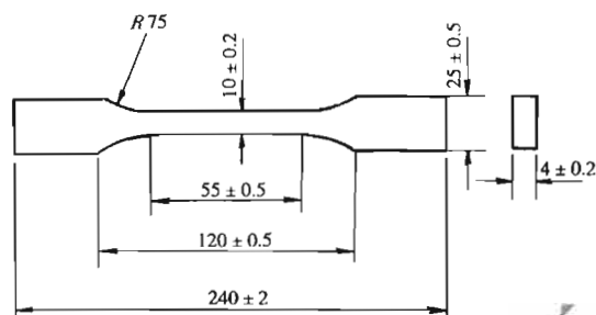
图 A.1.2-1 拉伸试样图(单位:mm)
