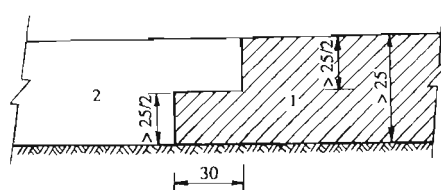
图 8.4.2 相错搭接法(单位:cm)
