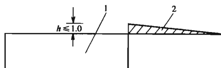
图 7.5.2 错台磨平法示意图(单位:cm)
