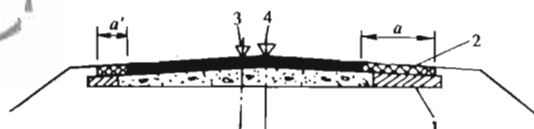
图 8.4.3-3 两侧不相等加宽路面
