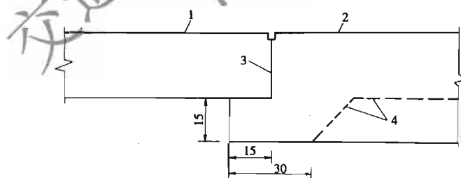
图 7.1.3-2 刨挖法(单位:cm)
