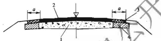
图 8.4.3-1 两侧相等加宽路面
