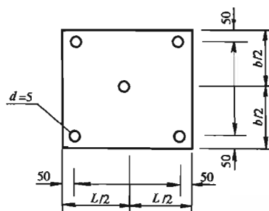
图 7.3.2 灌浆孔布置(单位:cm)
