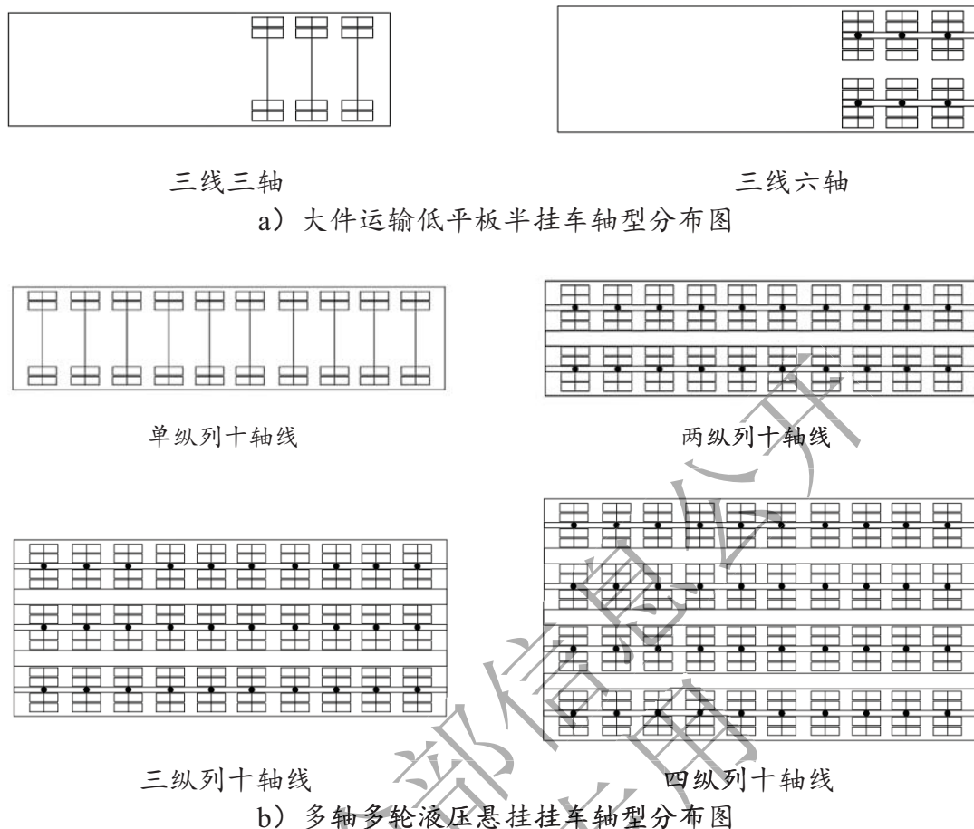
图 3-1 大件运输低平板半挂车和多轴多轮液压悬挂挂车的轴型分布图
