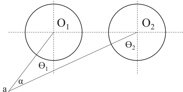
图 E.1.3-2 多个轴对称荷载下的主应力计算
