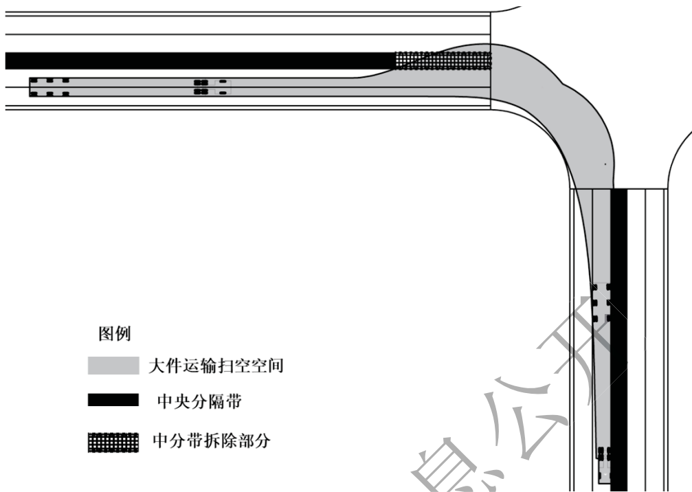
a) 拆除中央分隔设施
