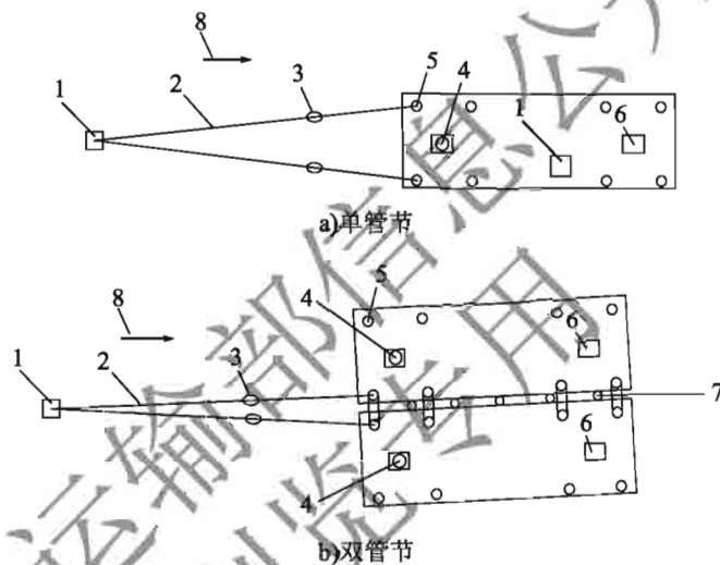
图 11-6 管节单点系泊示意图 1-锚块; 2-锚缆; 3-浮鼓; 4-人孔井; 5-系缆柱; 6-测量塔预埋件; 7-橡胶靠垫; 8-水流方向
