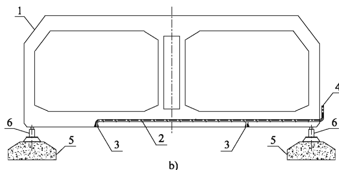
1-管节；2-灌砂管；3-灌砂管出口；4-灌砂管入口；5-临时支撑垫块；6-临时千斤顶
