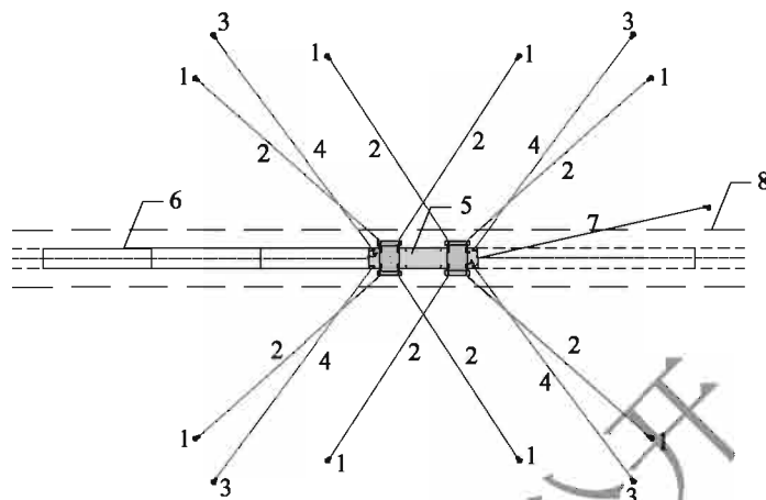
图 12-3 法向承力锚 (VLA) 块或大抓力锚方案系泊系统布置图
