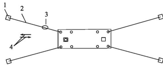
图 11-5 管节四点系泊示意图 1-锚块; 2-锚缆; 3-浮鼓; 4-水流方向
