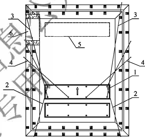
图 11-2 管节斜拉式横移示意图
