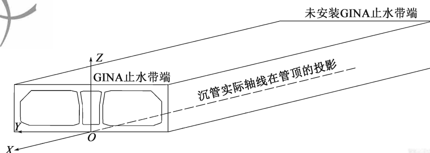
图 5-1 管节坐标系示意图
