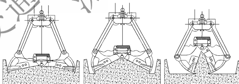
图 8-1 抓斗精挖功能原理示意图
