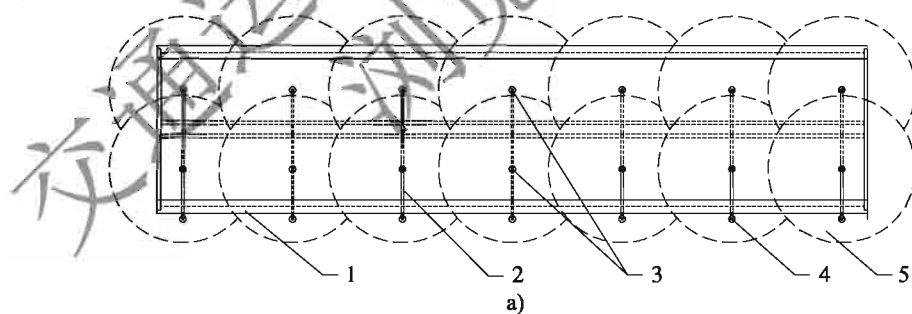
1-管节；2-灌砂管；3-灌砂管出口；4-灌砂管入口；5-砂积盘
