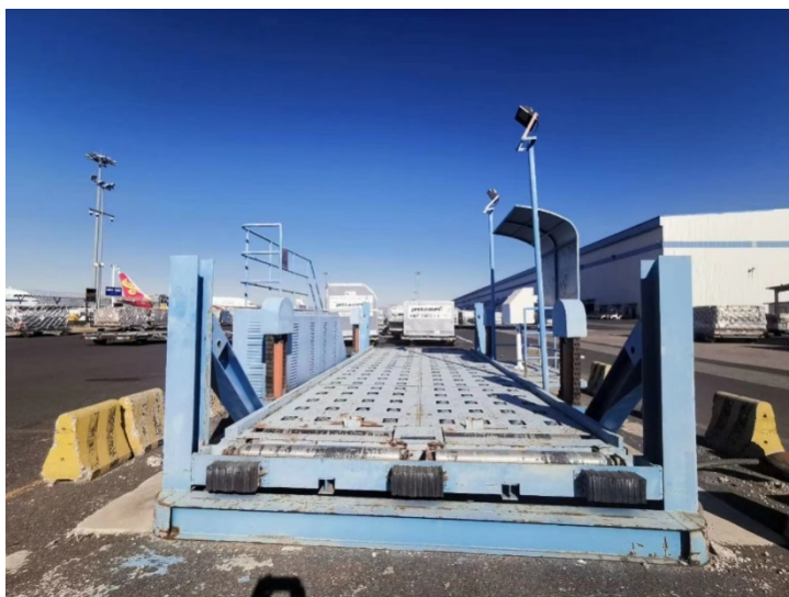
图 1 安装在首都机场货站的传送机
