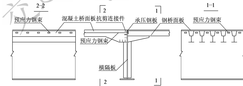
图 8.2.7 混合桥面板连接构造形式
