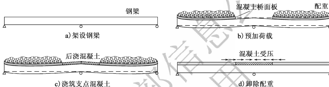
图 7.7.3-1 预加荷载法施加预应力
