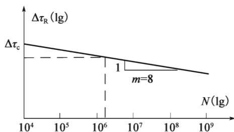
图 7-2 圆柱头焊钉剪应力疲劳细节曲线
