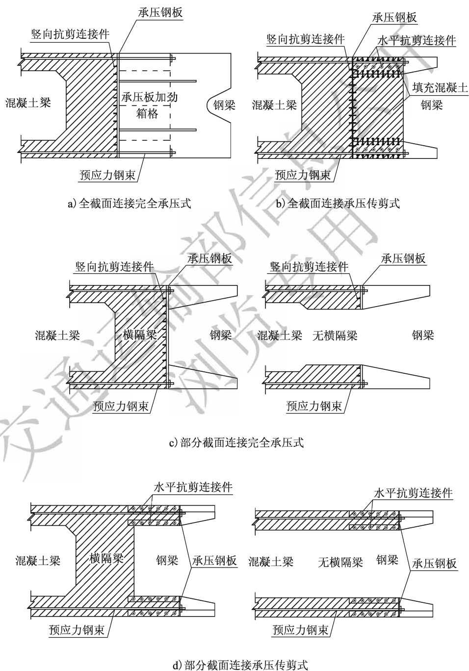
图 8.2.1 混合梁钢混连接形式
