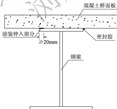
图 10.3.3 钢梁防腐涂装及密封示意图
