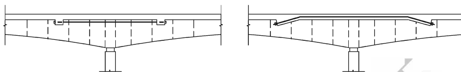
b) 连续组合梁桥负弯矩区施加预应力
