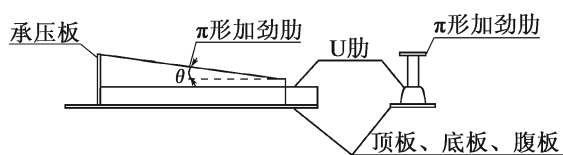
图 8.3.2-2 \pi 形加劲肋
