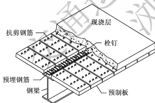
图 6-1 叠合板组合梁构造图
