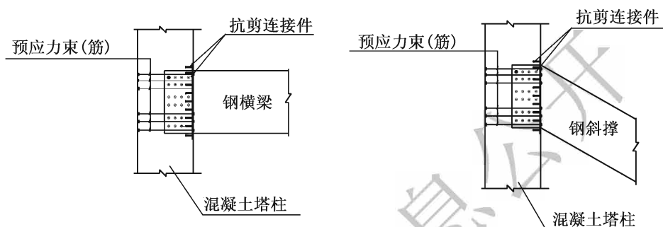
图 8.2.4 钢横梁（钢斜撑）与混凝土塔柱结合部连接构造示意图
