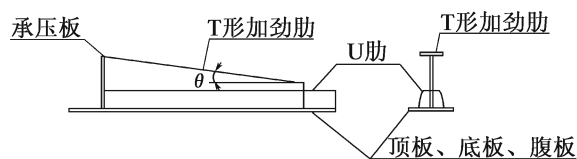
图 8.3.2-1 T 形加劲肋
