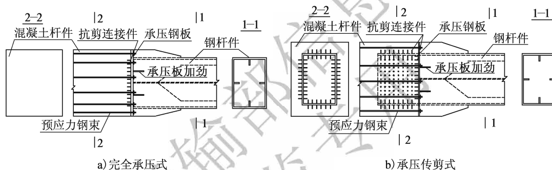
图 8.2.6 桁架混合杆件连接构造形式
