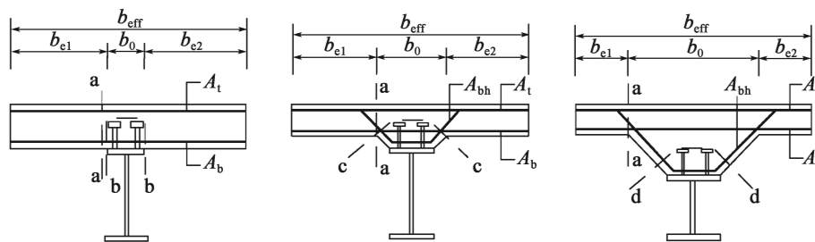
图 6.3.1 混凝土板纵向抗剪界面
