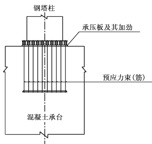
图 8.2.5-1 钢塔柱与混凝土承台完全承压式连接构造示意图
