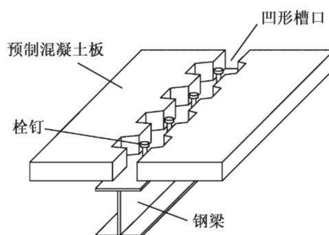
图 6-2 预制板组合梁构造图
