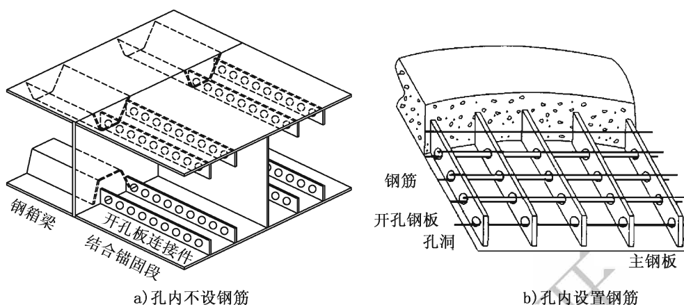
图 8.3.1 开孔板连接件形式
