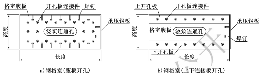
图 8.3.2-3 钢格室构造
