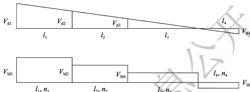
图 7-1 剪力分段示意图
