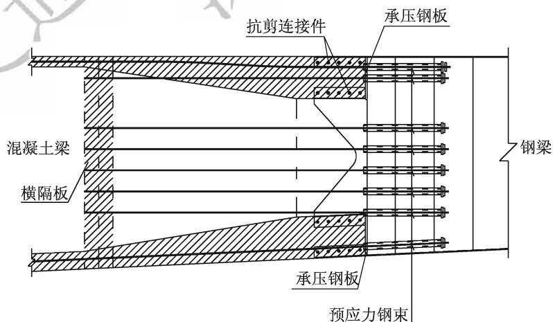
图 8-1 受弯为主的混合梁钢混连接构造
