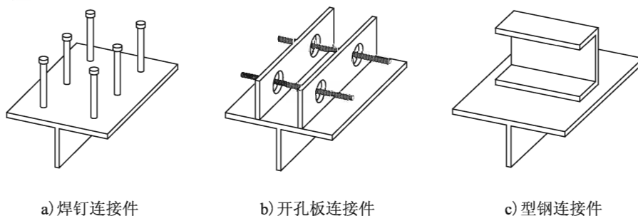
图9-1 常用连接件形式
