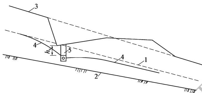
图 9.4.3 不透水层的横向坡度较陡时的渗沟流量计算 1-原地下水位;2-不透水层;3-坡面;4-设渗沟后地下水位;5-渗沟
