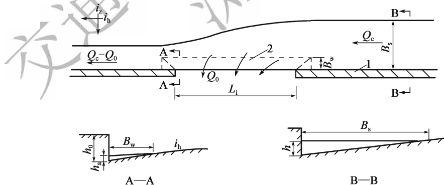
图 9.3.2 开口式泄水口周围的水流状况
