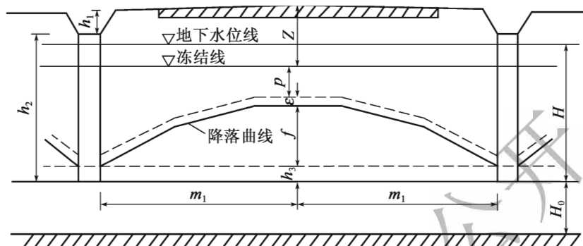
图 9.4.5 渗沟埋置深度计算
