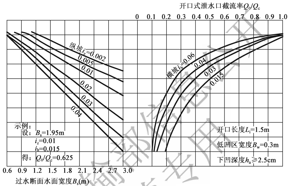
图 C-1 开口长度 L_1 = 1.5\text{m} , 低凹区宽度 B_w = 0.3\text{m} , 下凹深度 h_a \geq 2.5\text{cm}
