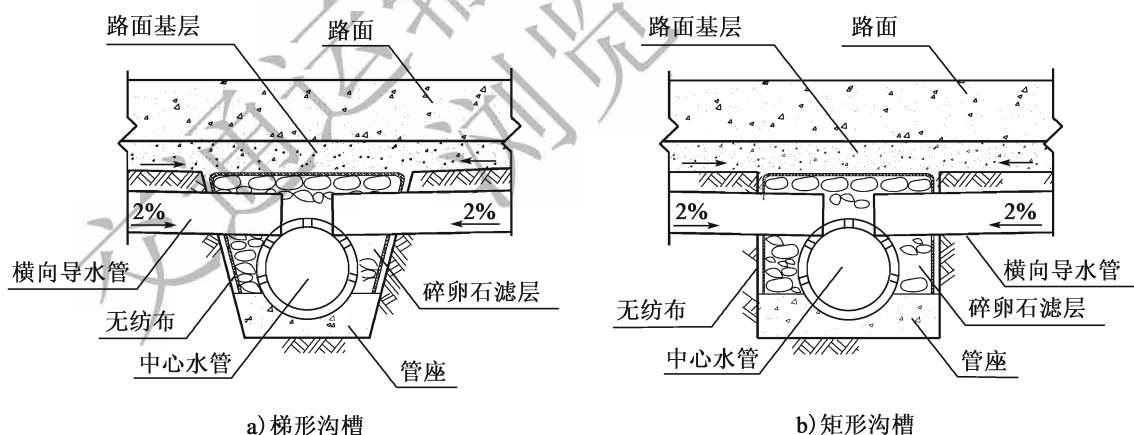
图 7.3.5-1 中心水沟
