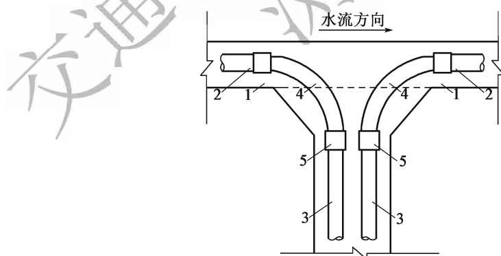
图 5.2.6 边缘排水系统出水管布置示意图
