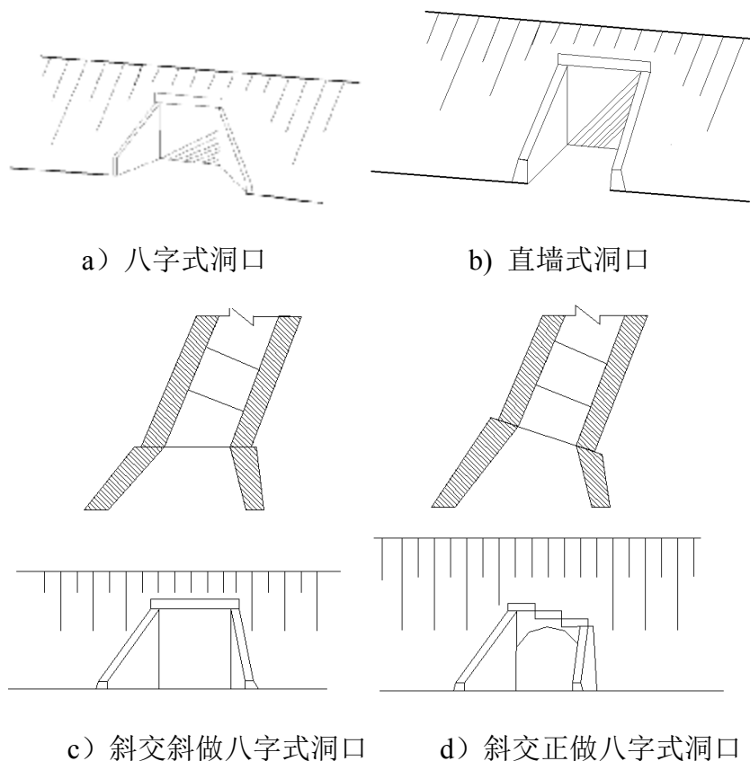
图 8.3.1 八字式洞口
