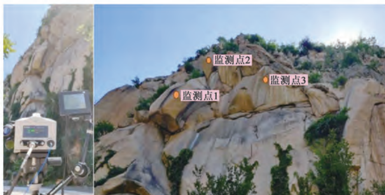
图 12 边坡预警系统和岩体监测
