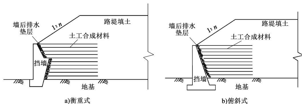
图 4.3.1-2 重力式挡墙墙后加筋结构形式
