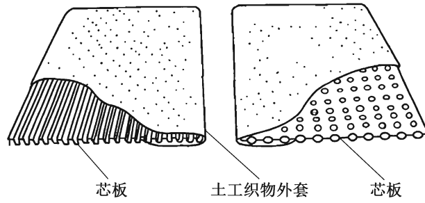
图 3-4 排水带典型断面
