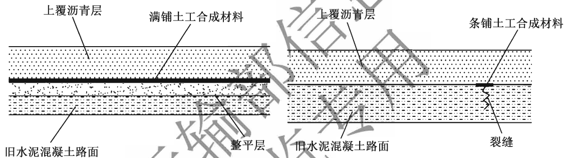
图 9.4.4-2 旧水泥混凝土路面加铺层结构示意图
