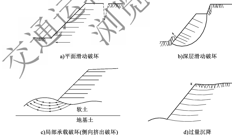
图 4-2 加筋路堤外部稳定破坏形式
