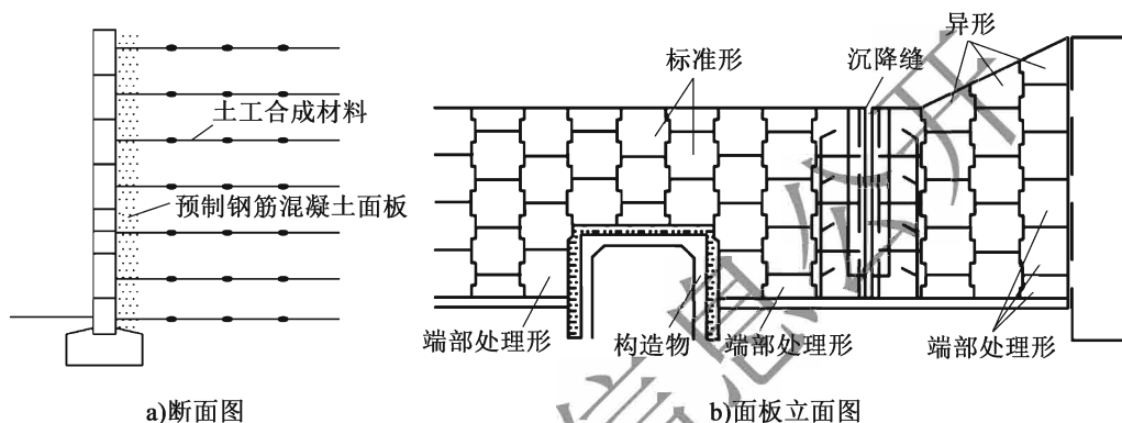
图 8.2.9 预制钢筋混凝土板块式墙面结构形式示意图
