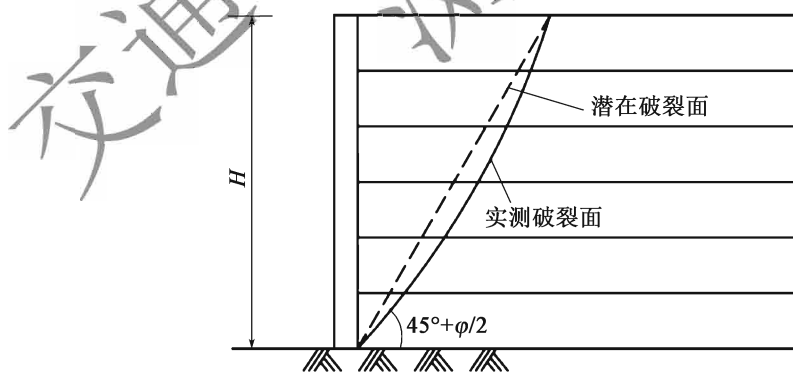
图 8-5 刚度较小的土工合成材料加筋土挡墙简化破裂面
