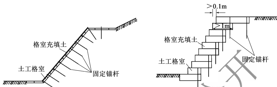
图 6.2.4 土工格室坡面生态防护结构形式
