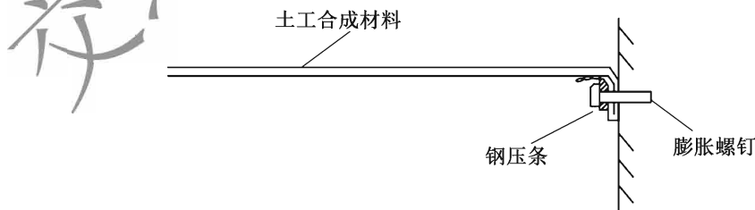
图 7.3.5-3 土工格栅与混凝土桥台连接示意图
