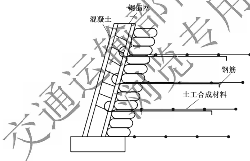
图 8.2.11 整体现浇钢筋混凝土墙面结构形式示意图
