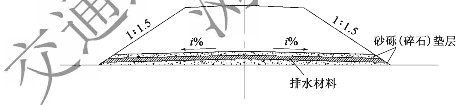
图 5.2.9 土工合成材料用于软弱地基顶部排水示意图
