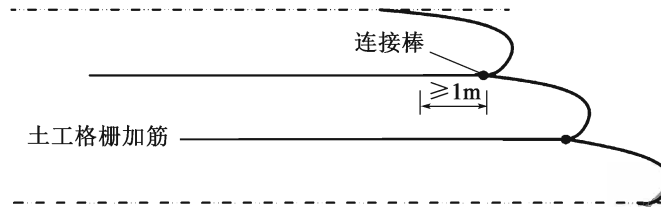
图 9.2.5-2 包边区土工格栅反包搭接示意图
