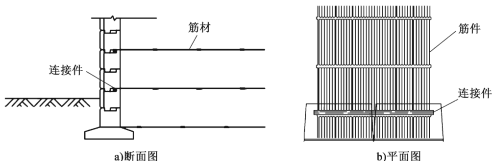
图 8-2 连接件连接示意图
