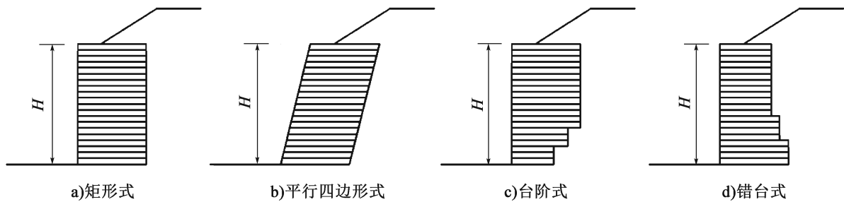
图 8.2.1 加筋土挡墙典型断面形式示意图
