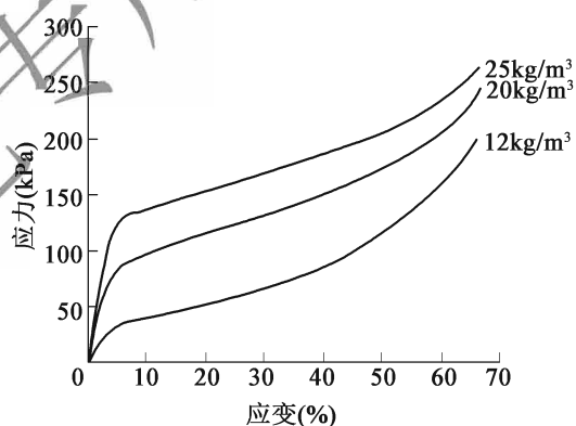
图 7-1 EPS 块单轴抗压应力-应变关系曲线
