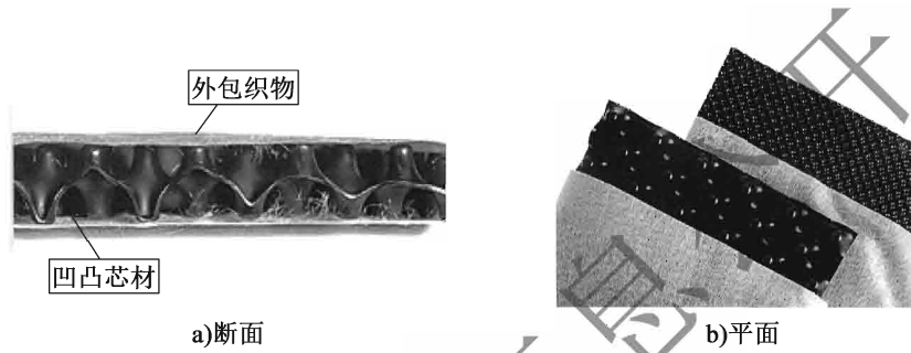
图 3-5 帽状芯材复合排水板
