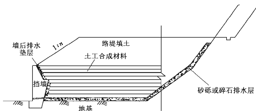
图 4.3.4 墙后加筋内部排水层设置示意图
