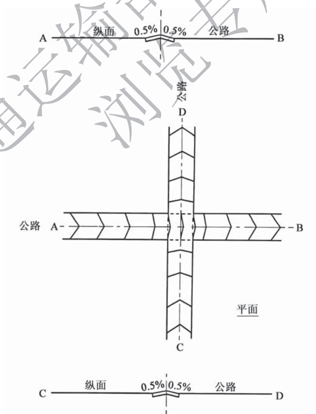
图 4.8.3 信号交叉或两功能相近交叉立面设计
