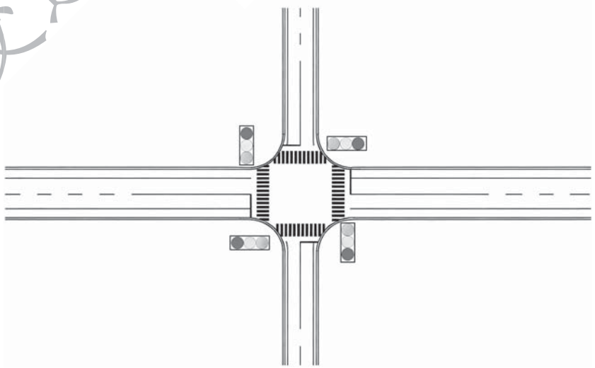
图 A.0.1-4 I 级平面交叉，十字，信号控制
