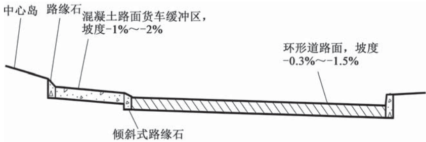
图 5.6.4 单坡型环形道 — 55 —
