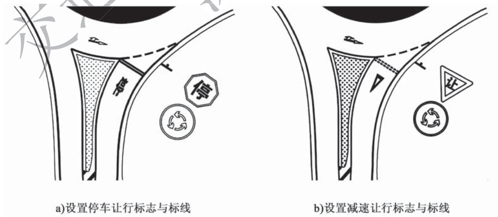
图 5.8.1-1 单车道环形交叉进口标志标线设置示意图
