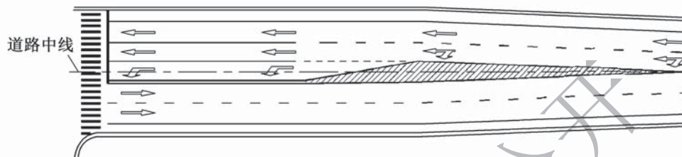
图 4.10.4-1 双侧偏移式左转弯车道
